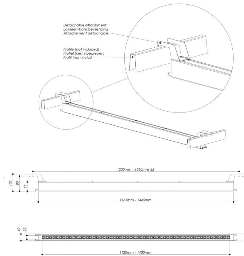
Dessin technique
