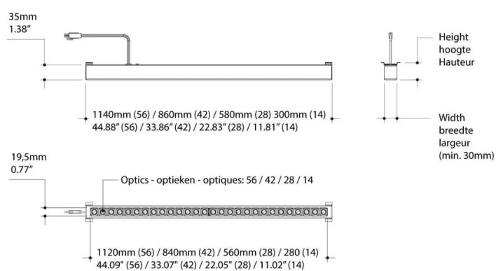
Dessin photométrique
