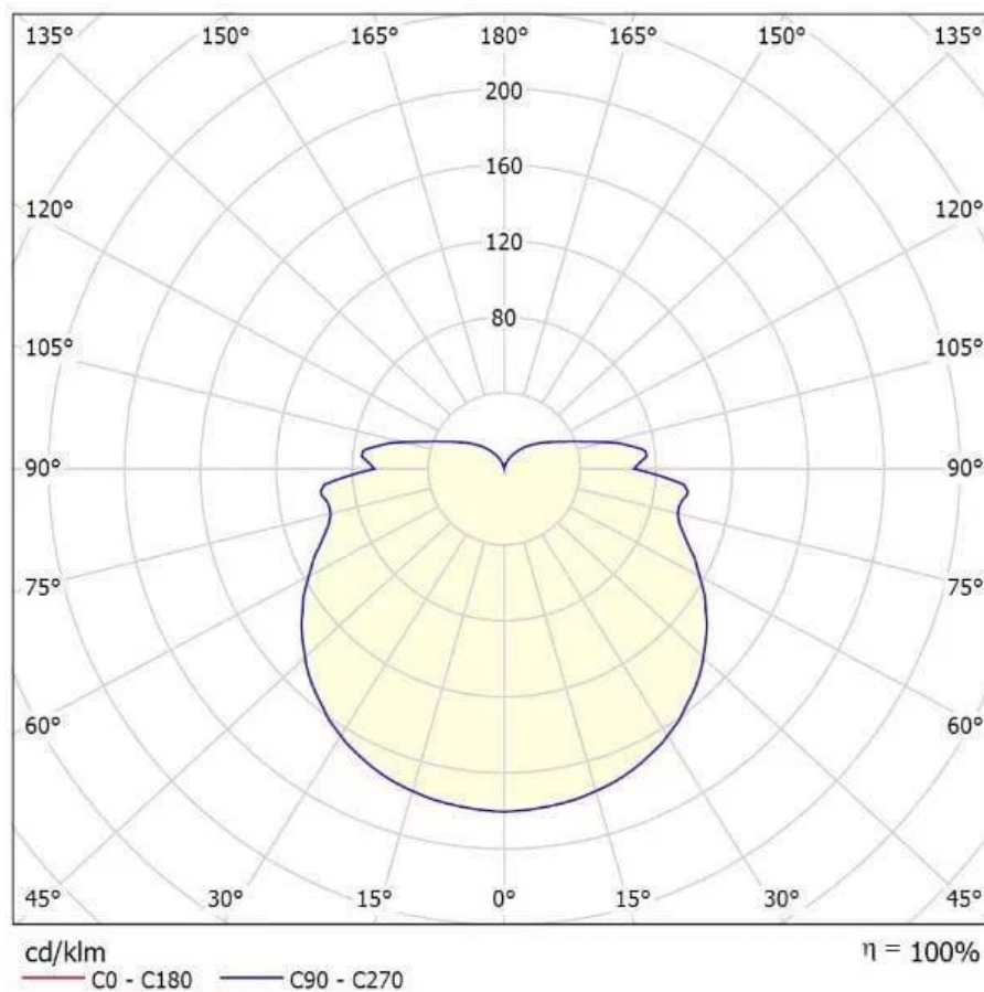
Dessin photométrique
