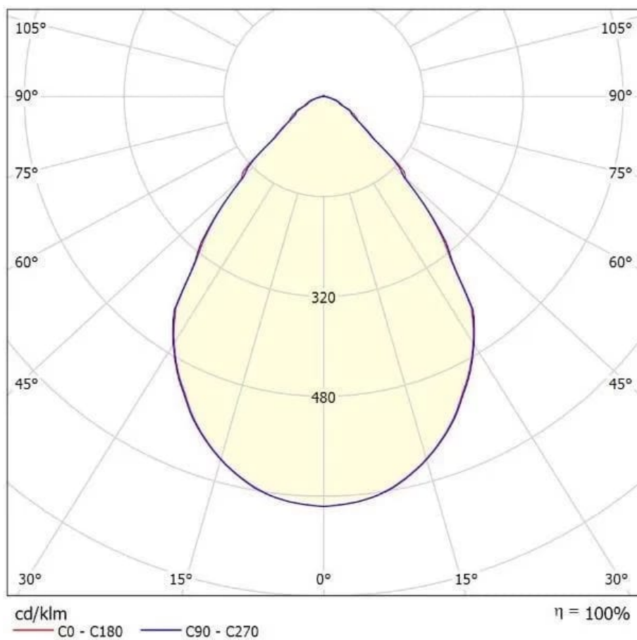
Lichttechnische tekening
